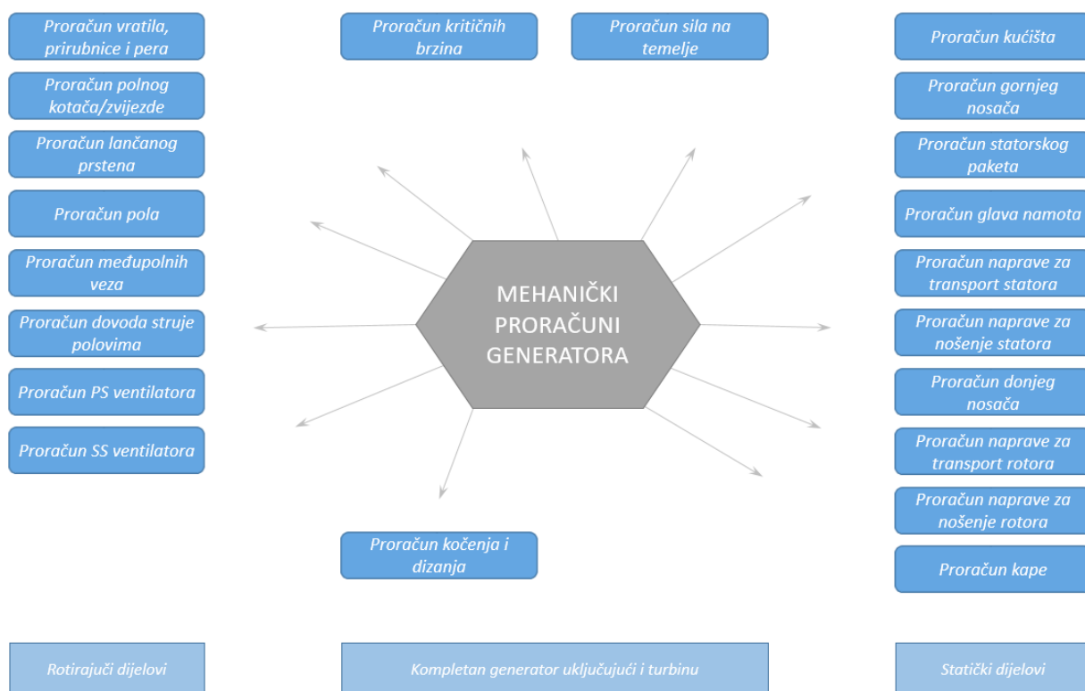
Slika 2.5. Uobičajeni mehanički proračuni za veliki generator prema [79]
