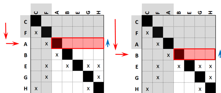
Slika I.II 2. korak topološkog particioniranja
