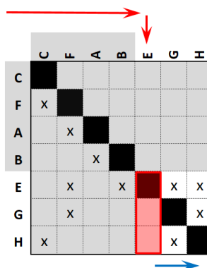
Slika I.III. 3. korak topološkog particioniranja
