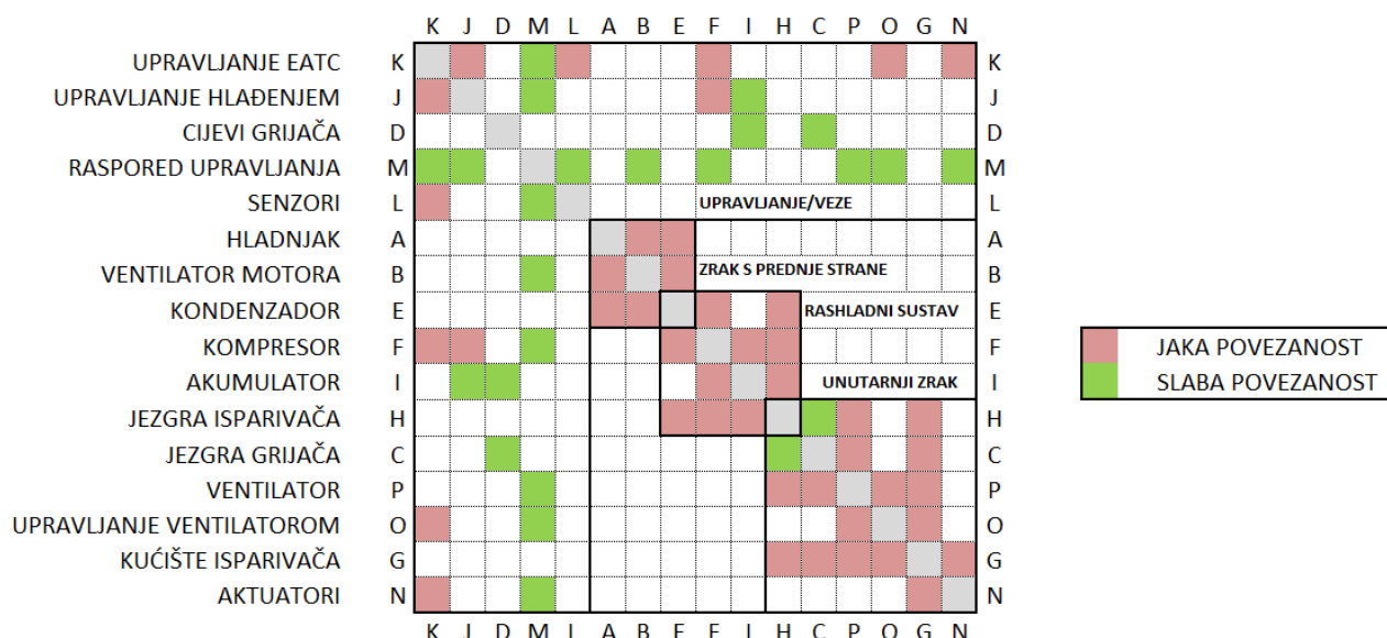
Slika 3.13. Particionirana DSM matrica kontrole klime u autu prema [25]
