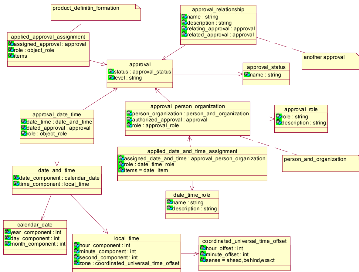
Slika 7-5 STEP struktura zapisa informacija o odobrenjima
