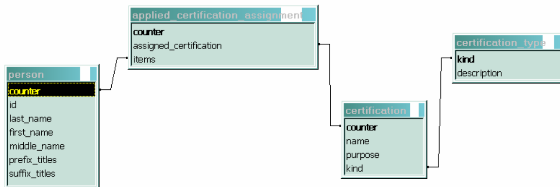
Slika 7-10 Struktura tablica i relacija za ovlasti
