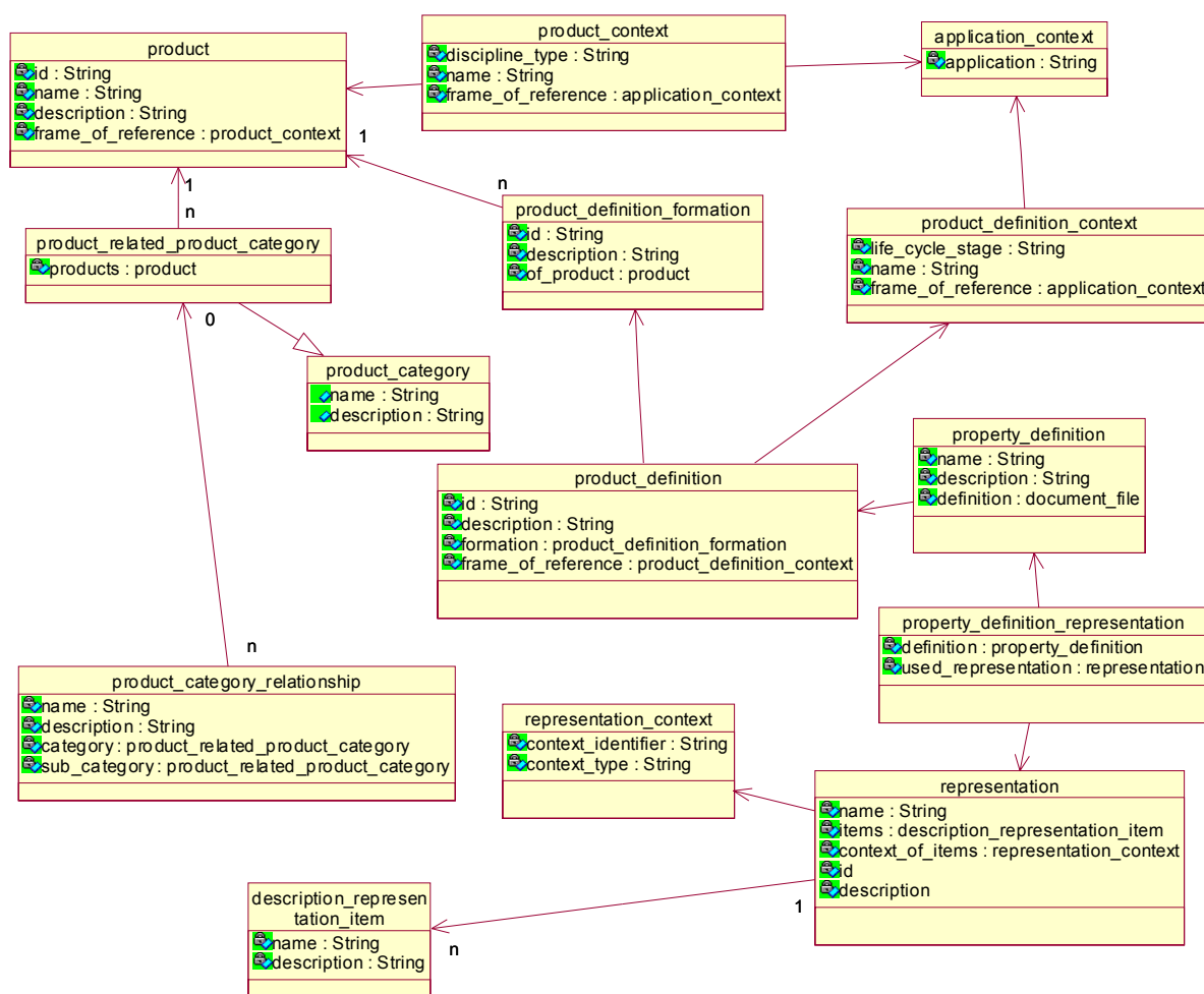
Slika 7-2 STEP Struktura zapisa konstrukcijskog znanja
