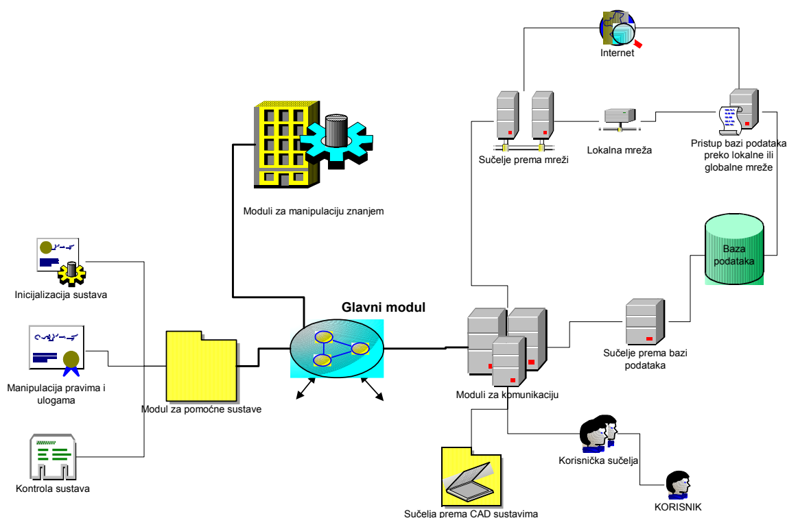
Slika 7-14 Struktura sustava za manipulaciju proširenim CAD modelom
