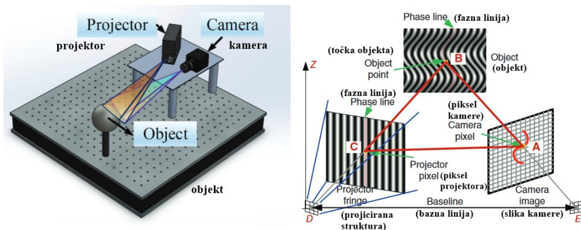
Slika 5. Ilustracija sustava za skeniranje structured light tehnologijom; shematski prikaz principa rada [13]
