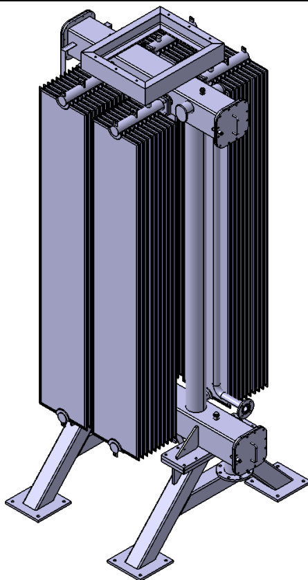
Slika 10.4 Varijanta 1 – izometrija
