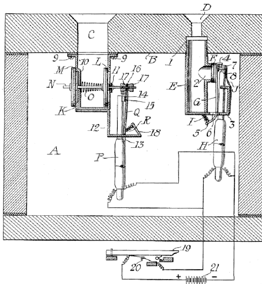
Slika 18. Patent US 1887076
