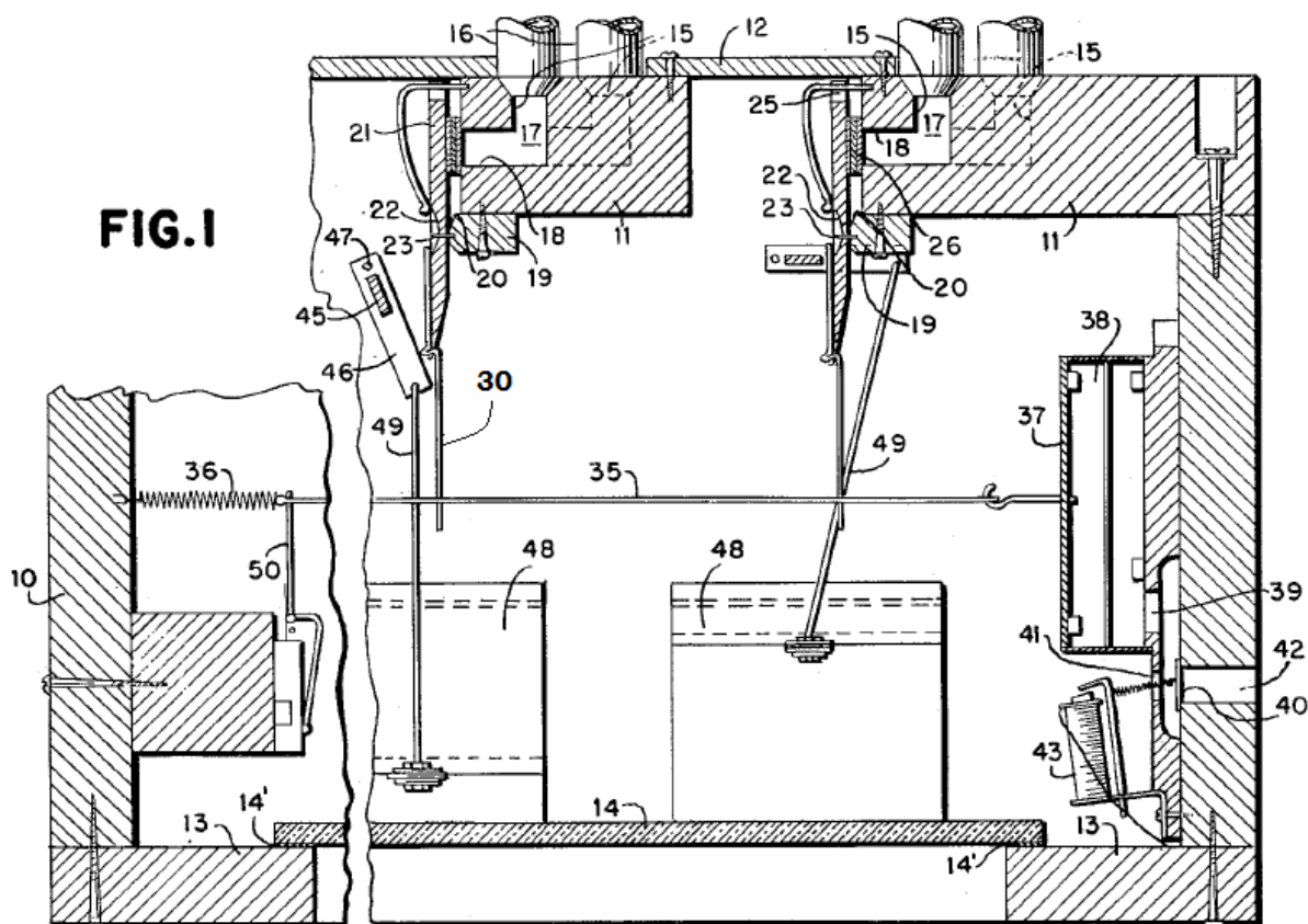
Slika 21. Patent US 2798399
