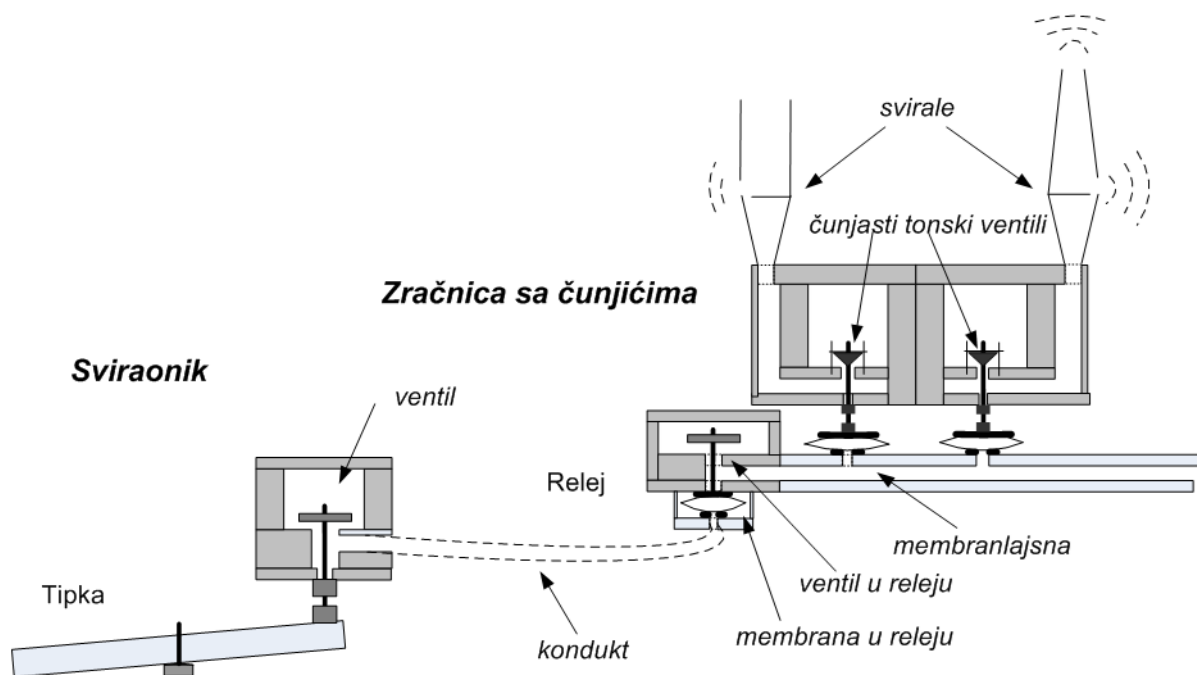
Slika 10. Prikaz rada pneumatskog sustava prijenosa na potisni zrak
