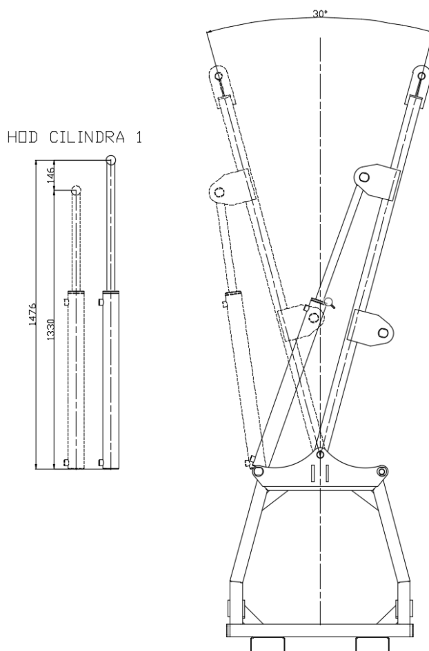
Slika 23. Hod cilindra 1
