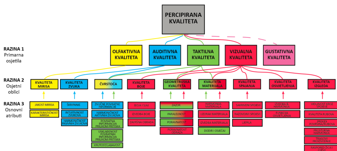
Slika 2 Struktura PQF-a [4]
