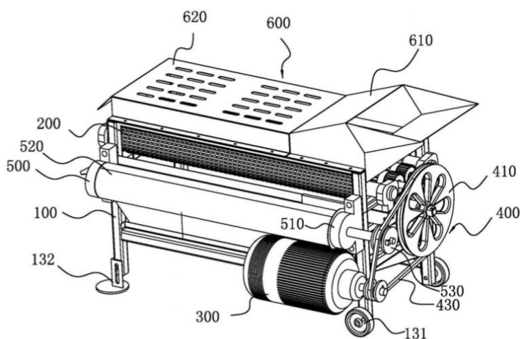
Slika 2.4. Patent CN107711057B [6]
