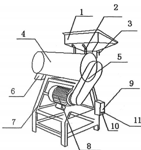
Slika 2.3. Patent CN202890418U [5]
