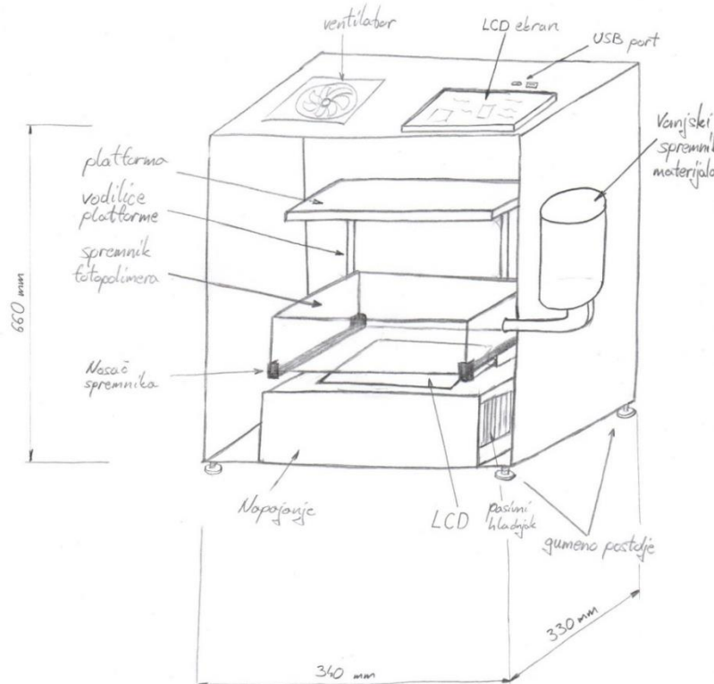
Slika 20 SLA uređaj [30]
