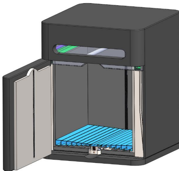
Slika 17 SLS uređaj [29]
