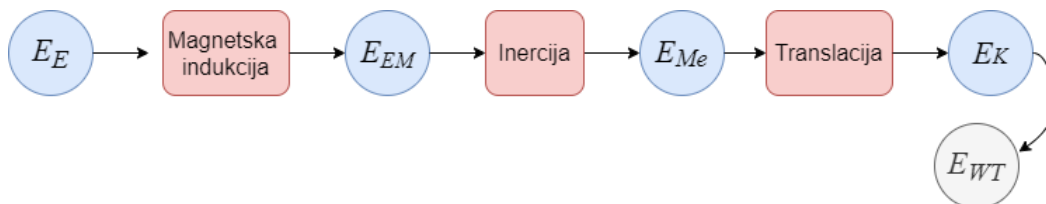
Slika 32 SLA- Lanac fizikalnih efekata L3a
