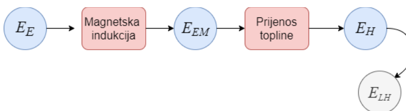
Slika 41 SLS - Lanac fizikalnih efekata L4
