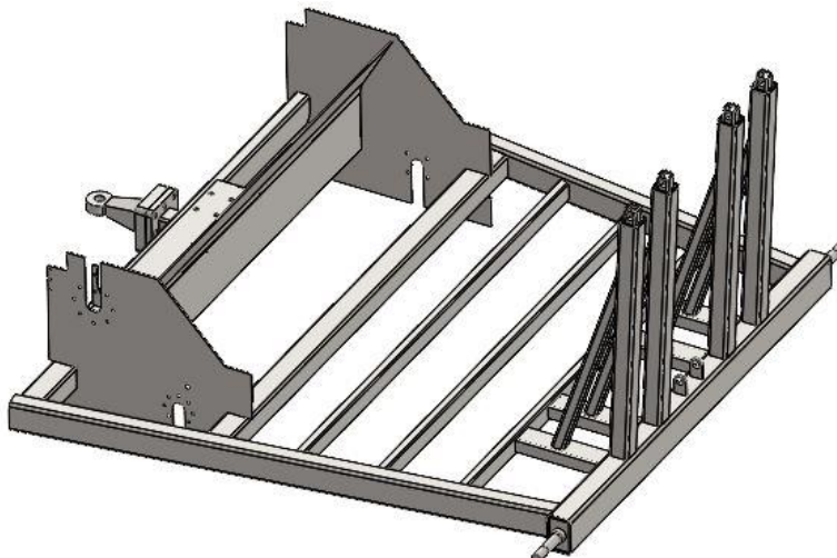
Slika 148. Nosiva konstrukcija
