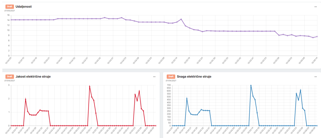
Slika 4.15. Vizualizacija podataka
