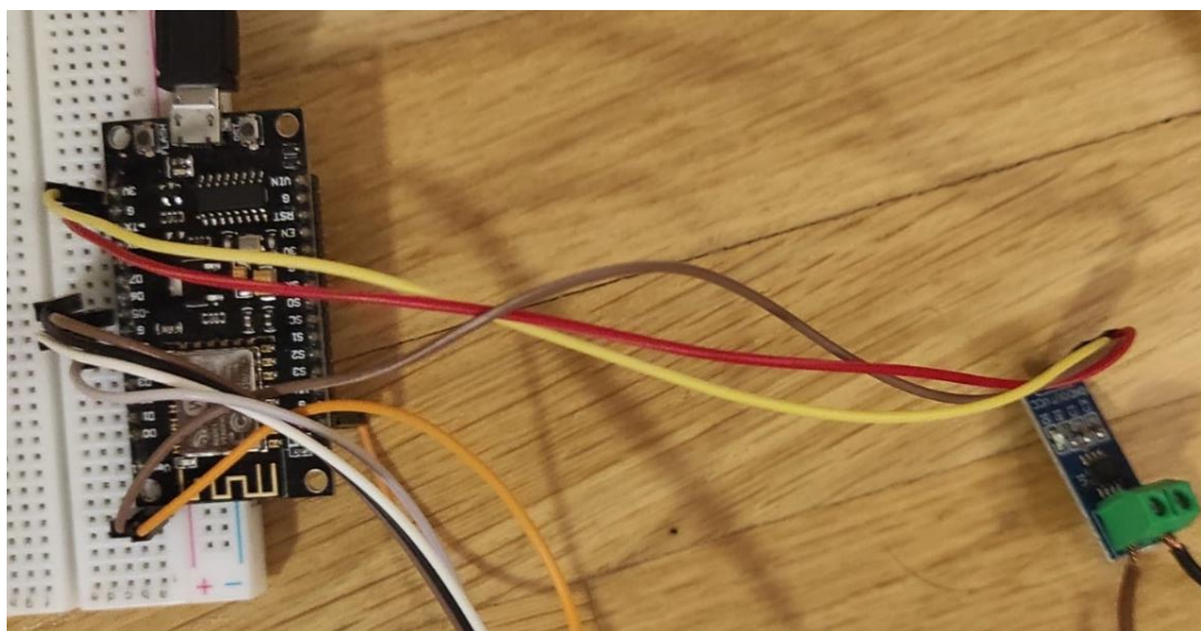
Slika 4.8. NodeMCU ESP8266 Wi-Fi modul (lijevo) i kablovi za spajanje sa senzorima
