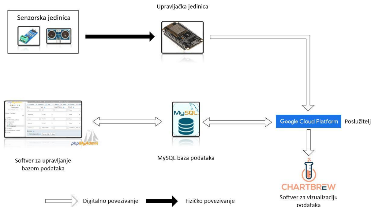
Slika 4.4. Shematski prikaz arhitekture digitalnog proizvoda sokovnika
