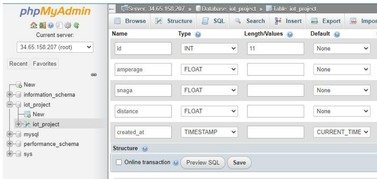
Slika 4.9. phpMyAdmin sučelje
