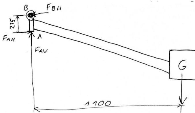
Slika 36. Model grede
