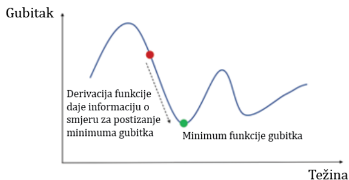
Slika 26. Primjer grafa funkcije gubitka, [35]
