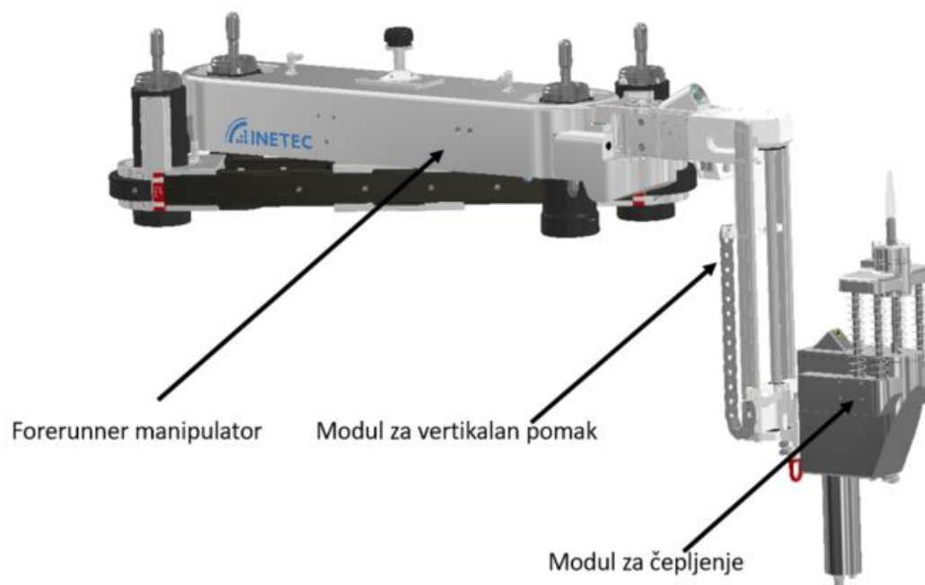
Slika 88. Modul za čepljenje s manipulatorom
