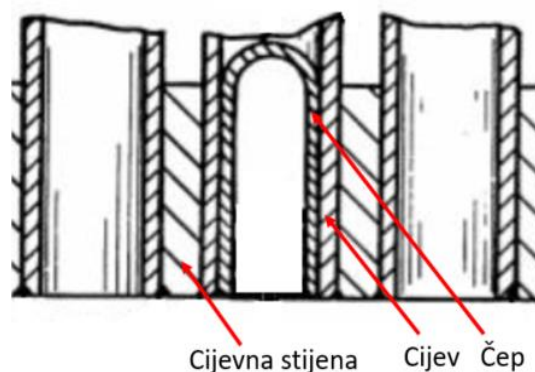
Slika 6. Začepljena cijev generatora pare [8]
